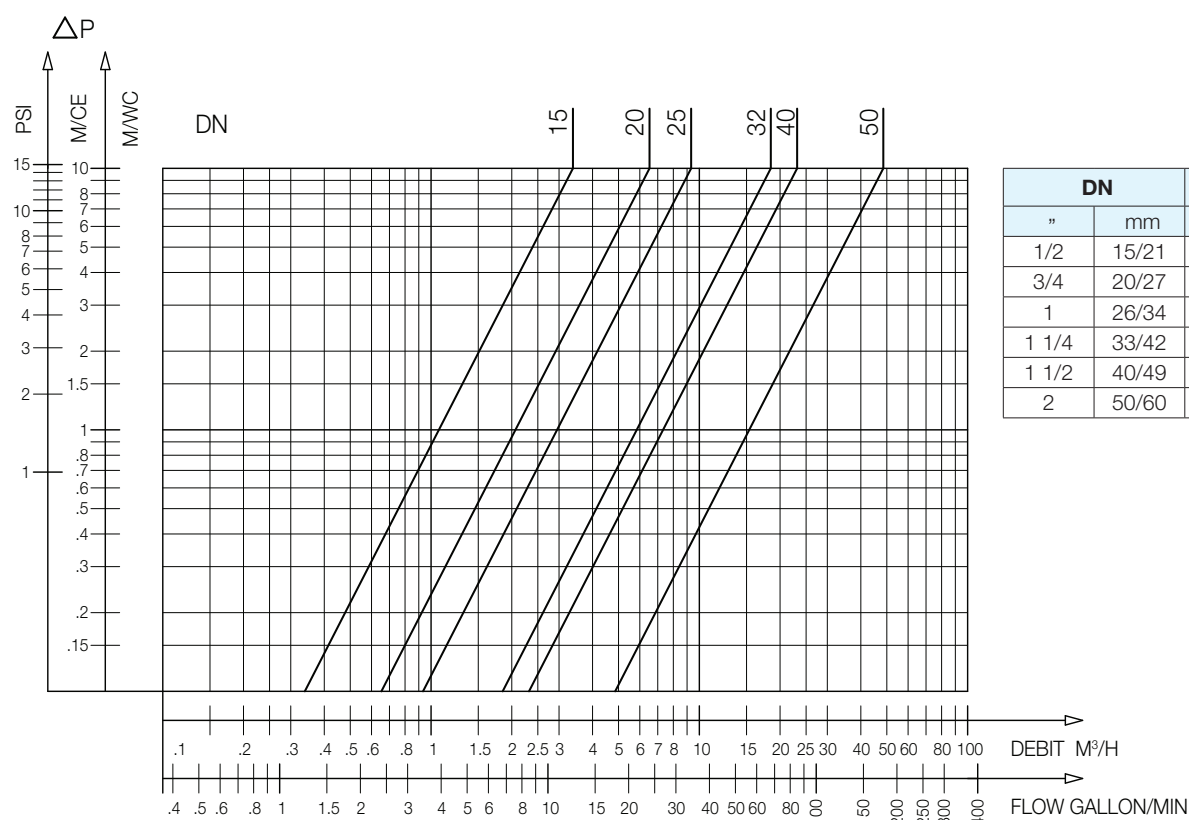
Y222 - Abaque des pertes de charge
