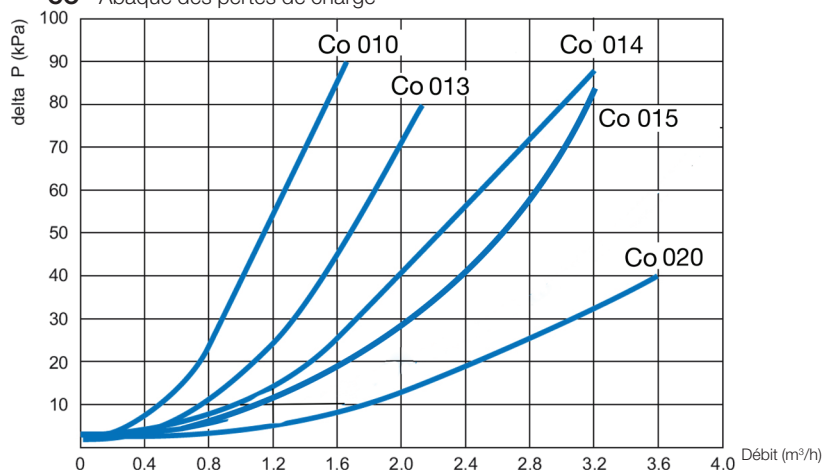
CO - Abaque des pertes de charge
