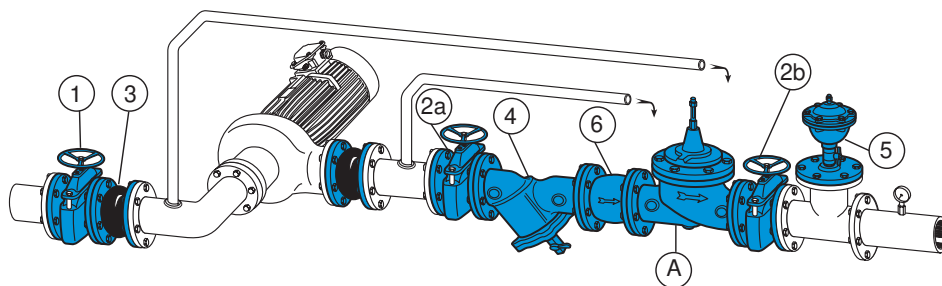
C 306 LI - Schéma d'installation de la vanne de régulation
