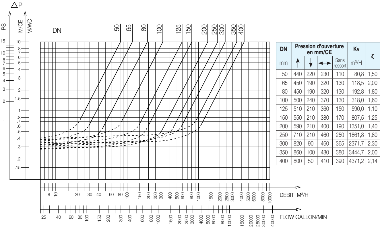
422 - Abaque des pertes de charge
