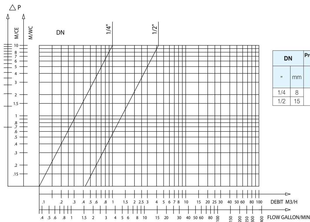
233X - Abaque des pertes de charge
